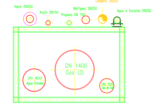
DISPOSICIÓN TIPO DE TUBERÍAS (Sección de celosías a LD-III)
