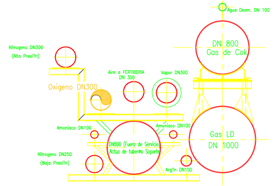
DISPOSICIÓN TIPO DE TUBERÍAS (Sección en Carretera Norte)
