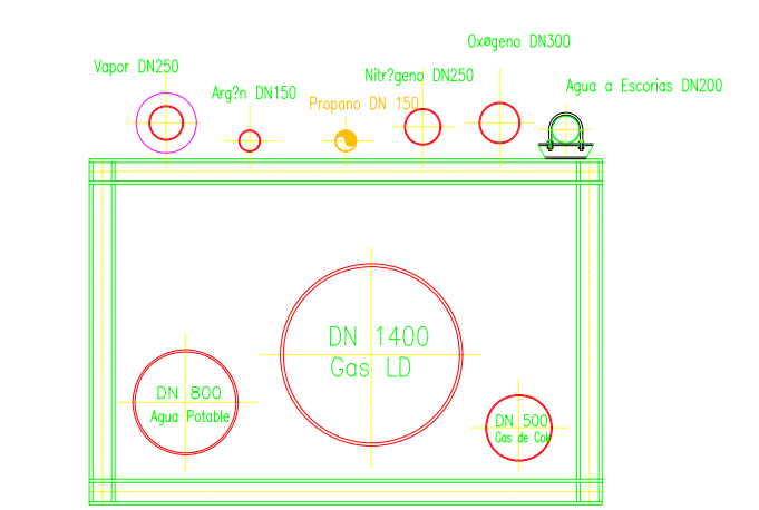
DISPOSICIÓN TIPO DE TUBERIAS (Sección de celosías a LD-III)
