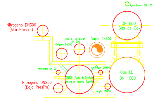
DISPOSICIÓN TIPO DE TUBERIAS (Sección en Carretera Norte)
