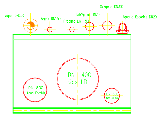
DISPOSICIÓN TIPO DE TUBERIAS (Sección de celosías a LD-III)
